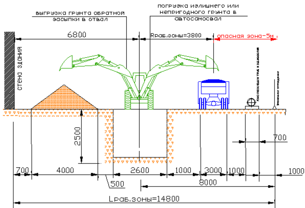
Рисунок 2.1 – Схема выбора экскаватора
