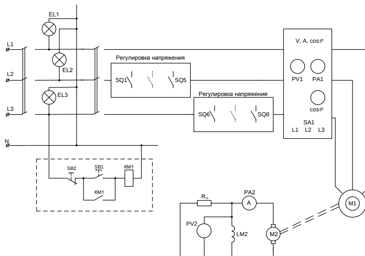
Рисунок 2.1 – Принципиальная схема стэнда
