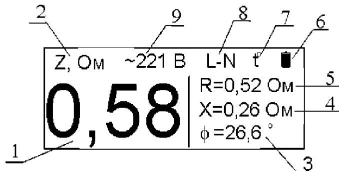
Рисунок 8.3 – Вид индикатора в режиме «фаза-нуль»:
