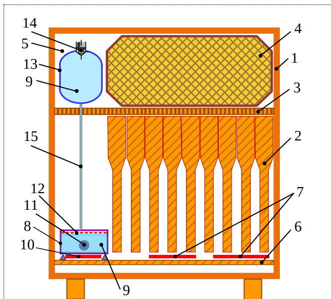
Рисунок 1 – Разрез улья с конструктивными элементами
