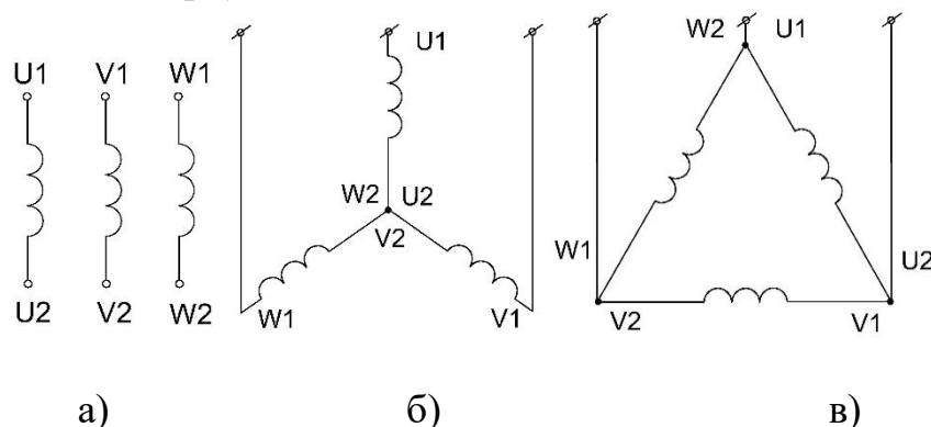
Рис 1.1 Маркировка выводов обмоток асинхронного двигателя (а) и схемы соединения «звездой» (б) и «треугольником» (в)
