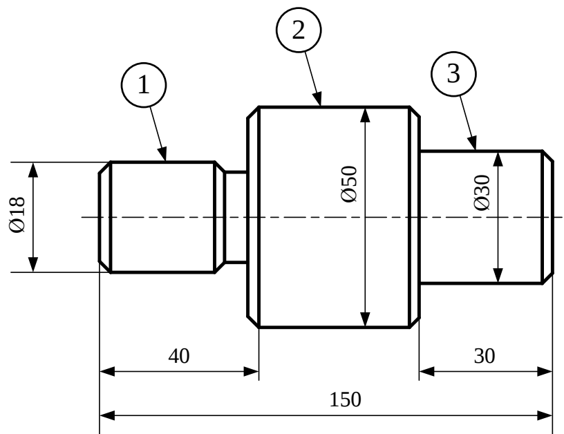
Рисунок 1 – Эскиз детали
