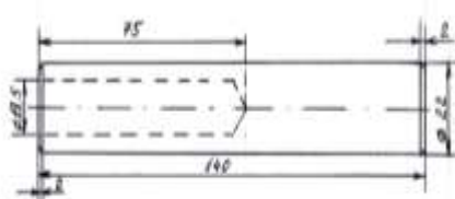
Рисунок 1 – Изготовление навеса
