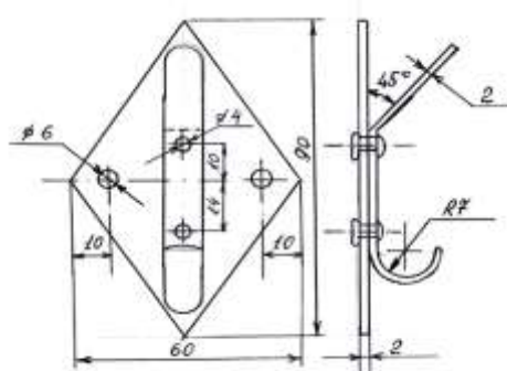
Рисунок 1 – Изготовление вешалки
