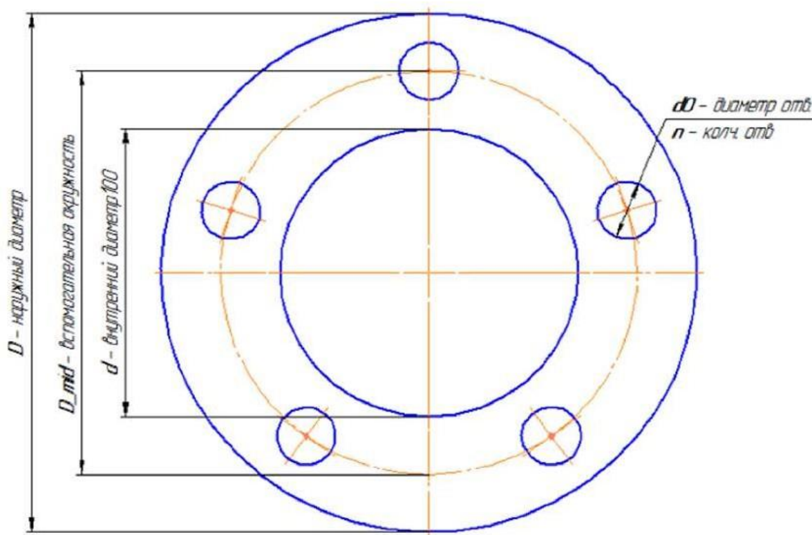
Рисунок 1 Фланец
