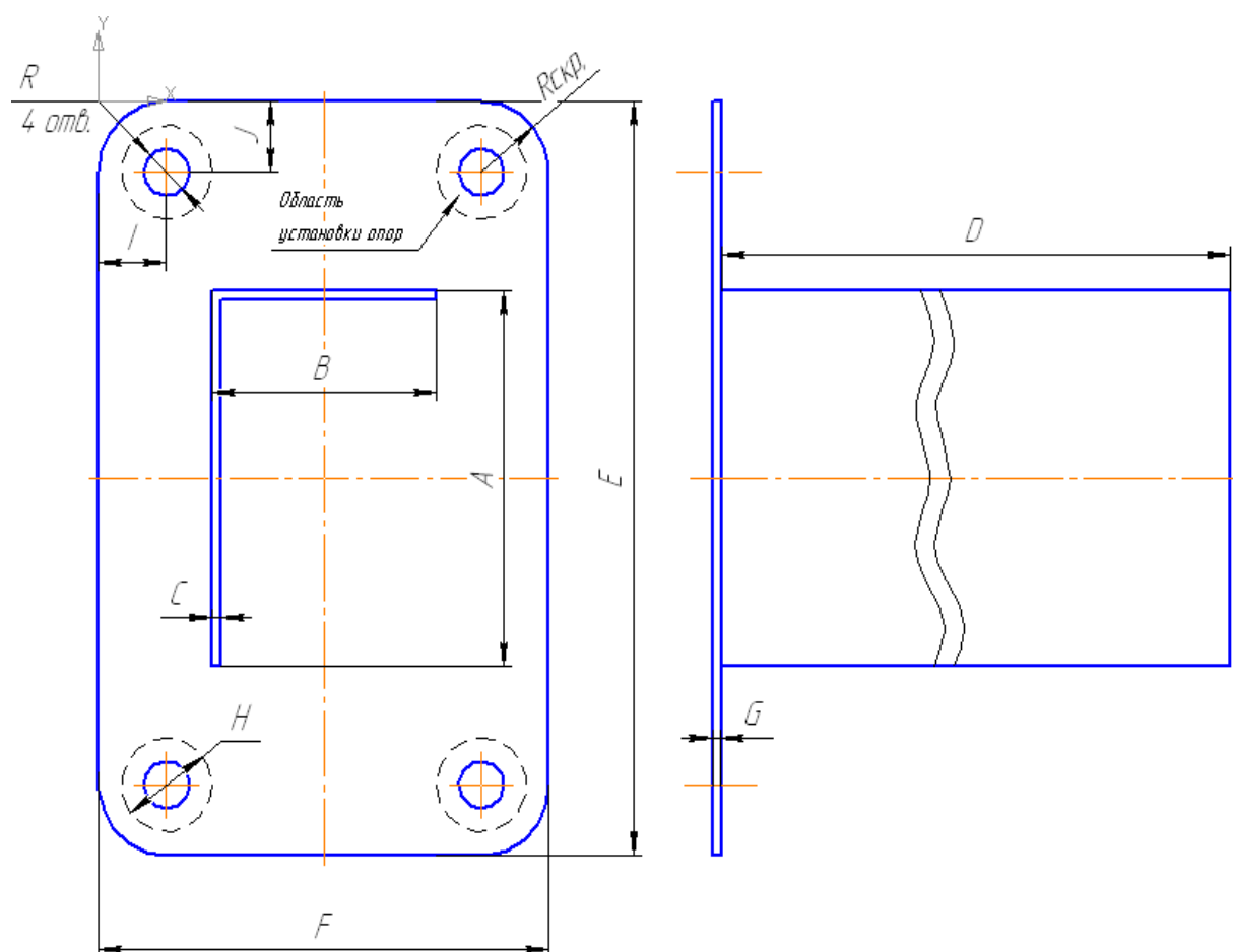
Рисунок 2 Чертёж кронштейна для самостоятельного выполнения расчёта.
