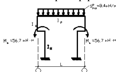
Рис.2.3 – Расчетная схема рамы от действия снеговой нагрузки (нагрузка № 2)
