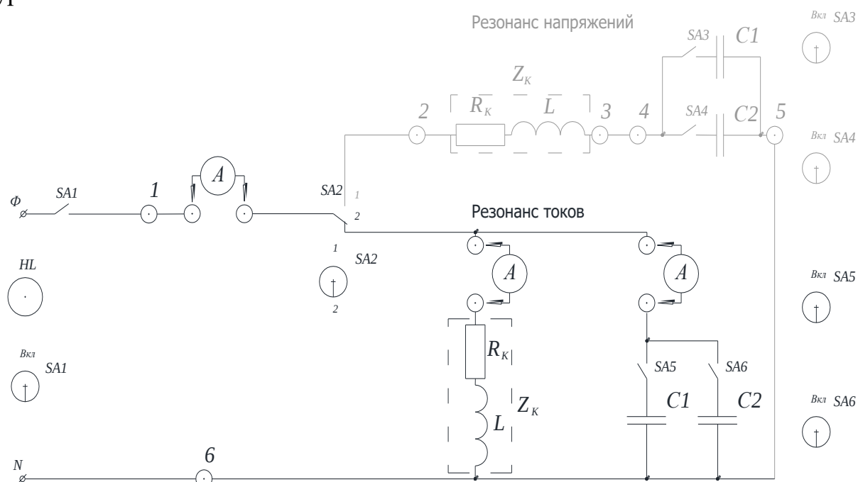
Рисунок 4.2 – Исследуемая схема
