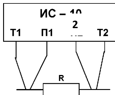
Рисунок 4.1 – Схема подключения при четырехпроводном методе измерения Измерение сопротивления металлосоединений защитных проводников трех- проводным методом
