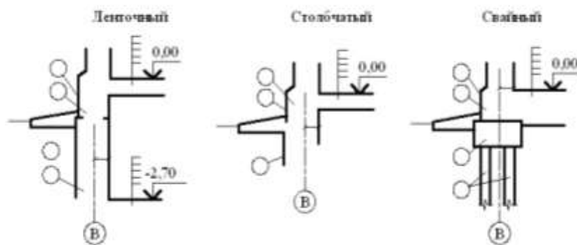
Варианты сечения 2-2
