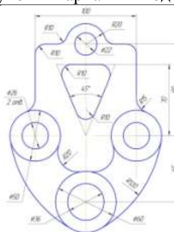
Рисунок 4 Вариант 4 Подвеска
