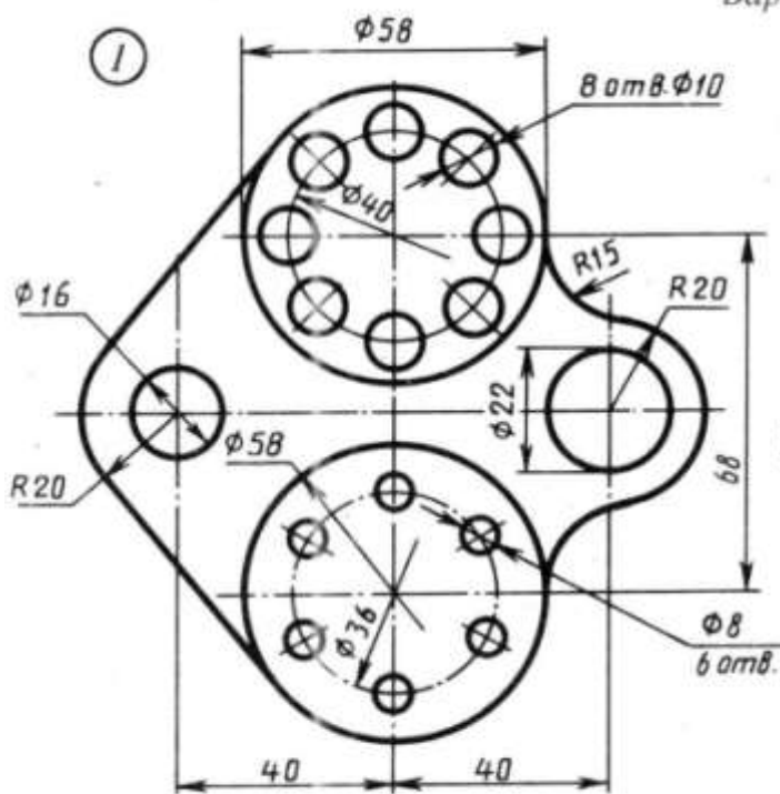
Корпус
