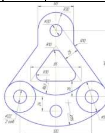
Рисунок 6 Вариант 6 Подвеска
