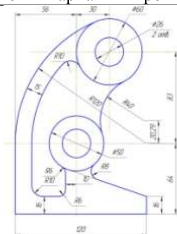
Рисунок 3 Вариант 3 Станина
