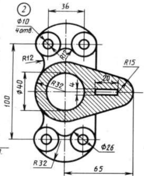
Кронштейн
