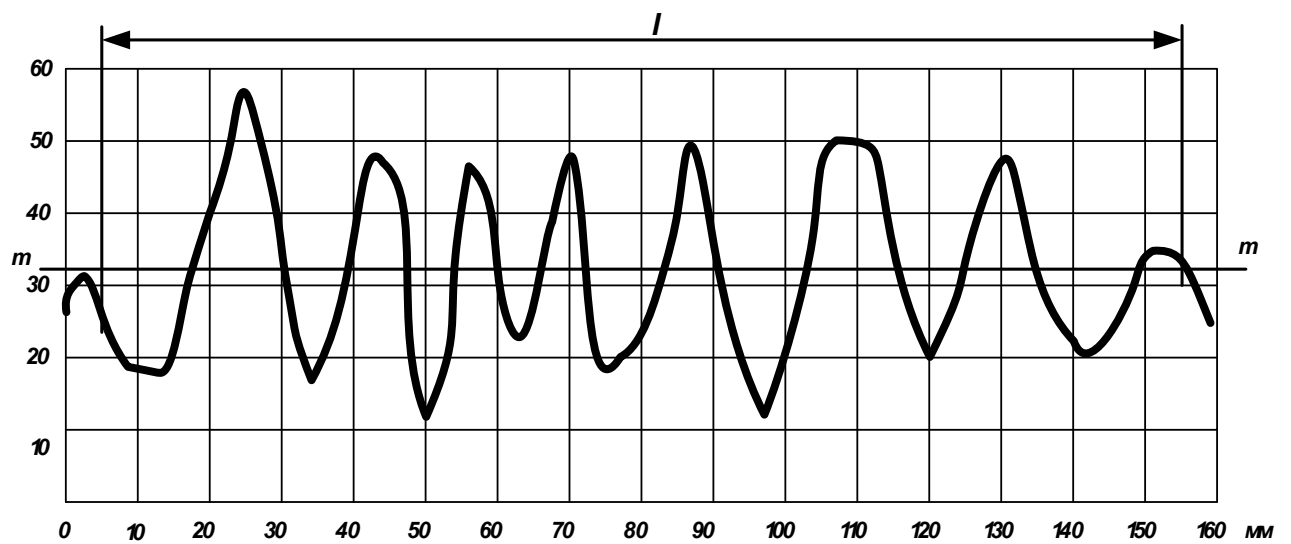
Рисунок 3.21 – Варианты 15, 30, 45, 60, 75 для задания № 1
