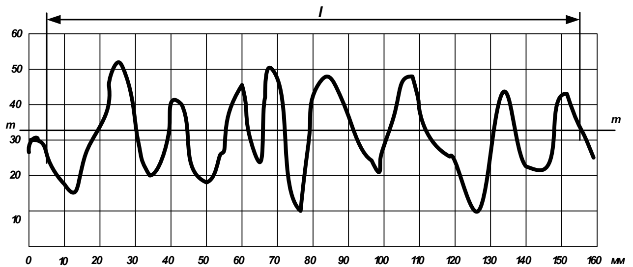
Рисунок 3.12 – Варианты 6, 21, 36, 51, 66 для задания № 1
