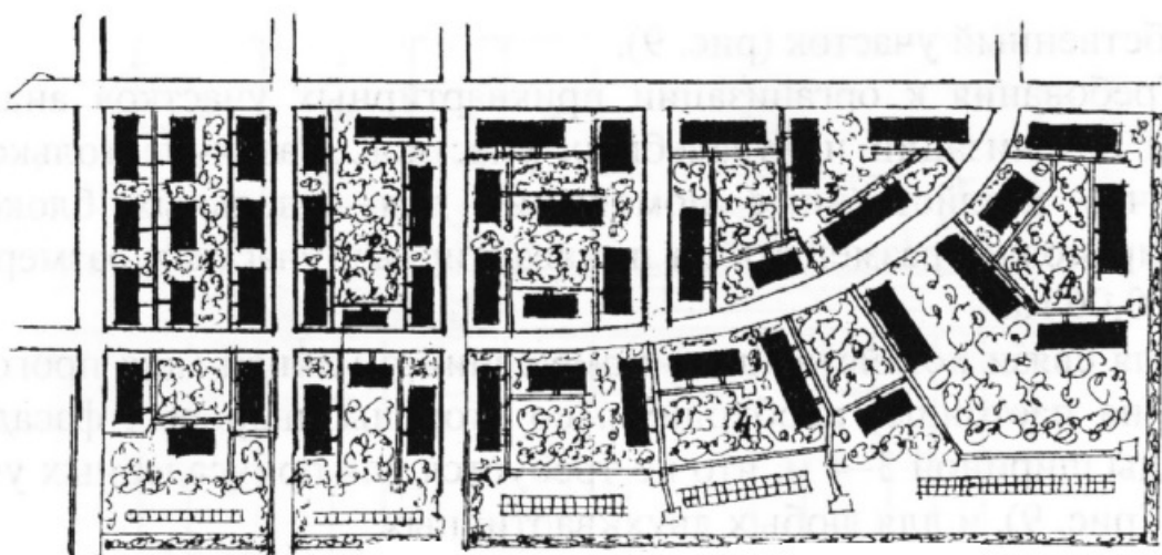
Рисунок 9 – Приемы застройки жилых территорий секционными домами
