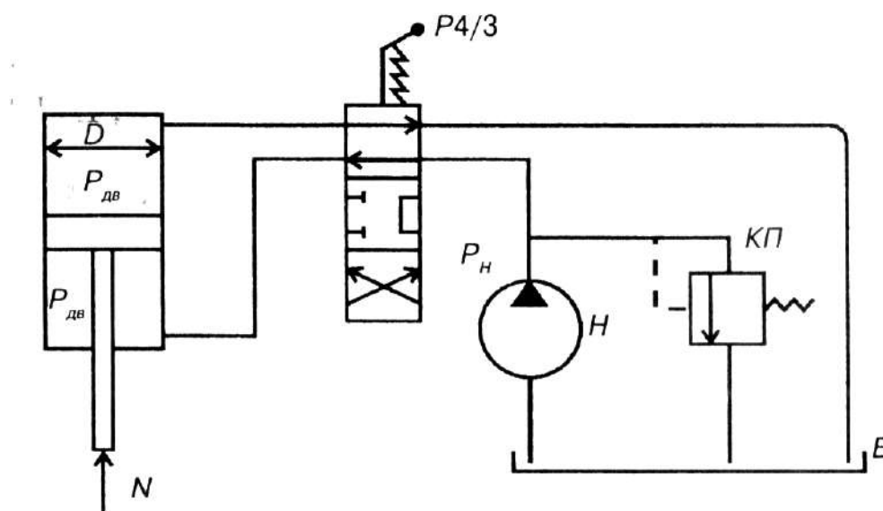
Рисунок 1 – Схема объемного гидропривода возвратно-поступательного движения
