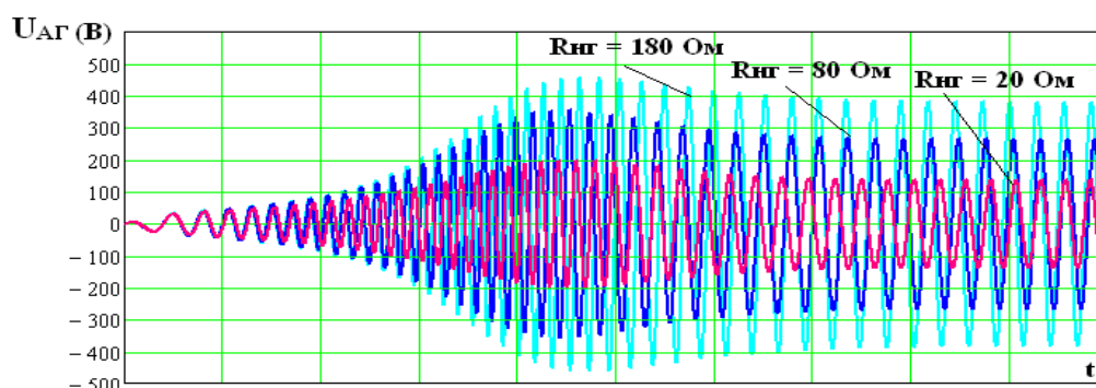
Рисунок 2.6 – Модель самовозбуждения АГ с линейной L_m при разных R_{нр}
