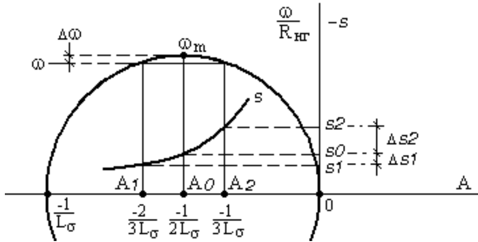
Рисунок 2.5 – Анализ устойчивости режимов работы АГ
