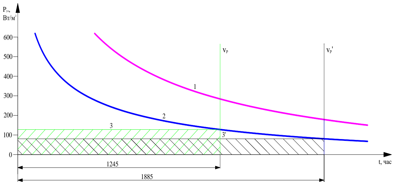
Рисунок 1.6 – Распределение удельной мощности ветра на высоте 10 м: 1 – теоретическое распределение удельной мощности ветрового потока; 2 – удельная мощность на валу ветроколеса; 3 и 3' – фактическая удельная мощность ветроэнергетической установки
