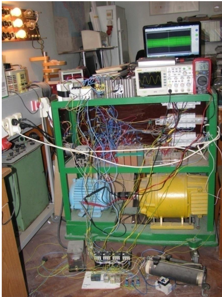
Рисунок 4.3 – Внешний вид испытательного стенда
