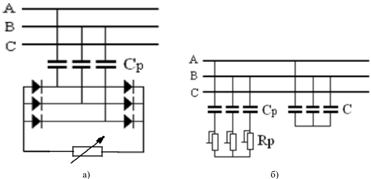
Рисунок 3.2 – Применяемая (а) и эквивалентная (б) схемы
