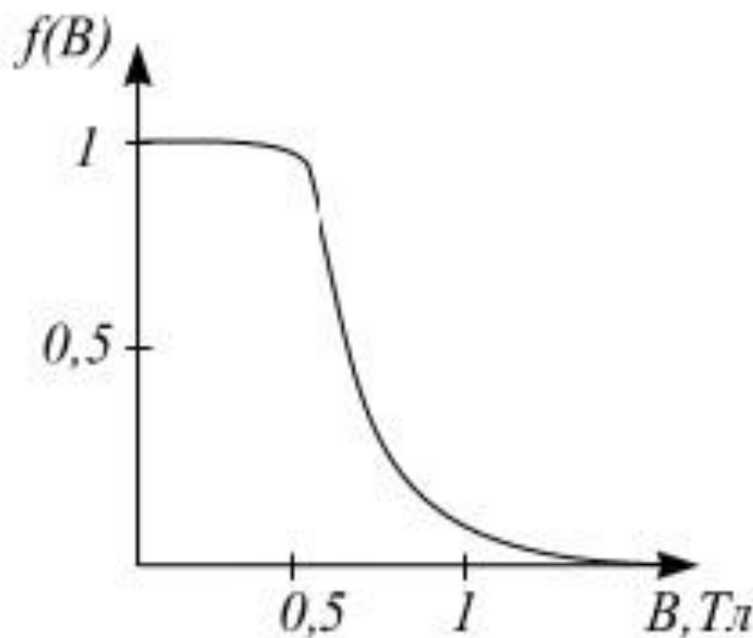
Рисунок 1.19 – Функция уменьшения магнитной связи между обмотками АГ
