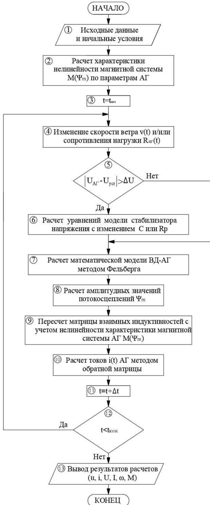
Рисунок 3.4 – Алгоритм решения уравнений модели «ВД-АГ-нагрузка» со стабилизатором напряжения для расчета параметров и режимов работы ВЭУ
