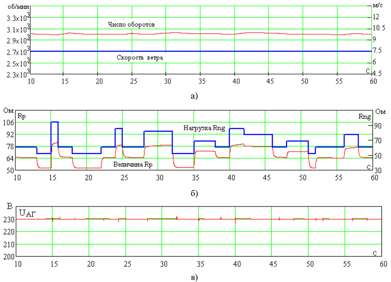
Рисунок 3.14 – Результаты моделирования работы системы ВД-АГ-нагрузка со стабилизатором напряжения при переменной нагрузке и постоянной скорости ветра с регулированием тока возбуждения: а – скорость ветра и число оборотов АГ, б – величина емкости возбуждения и величина нагрузки АГ, в – напряжение на выводах АГ
