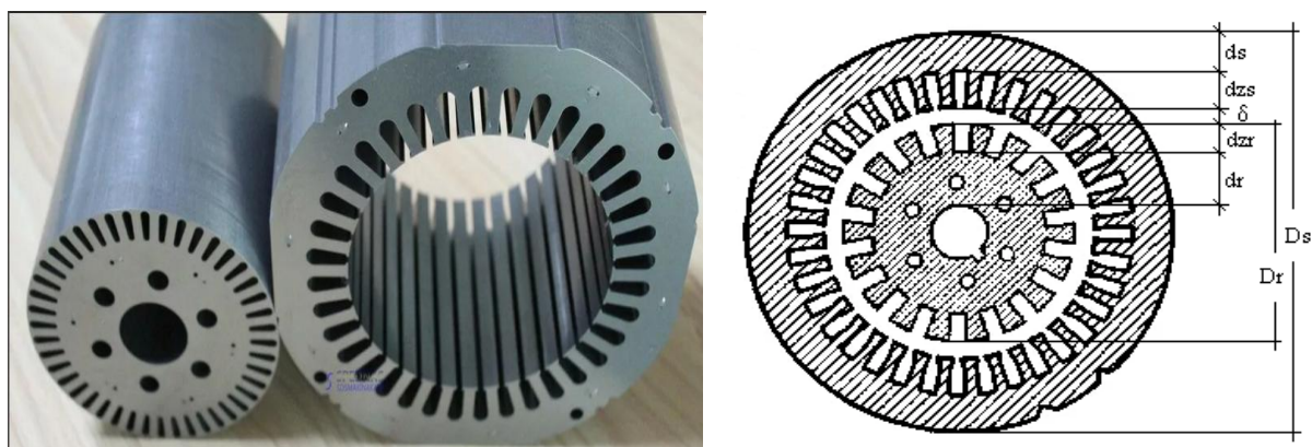
D_{si} , D_r – внешние диаметры статора и ротора, d_s и d_r – толщина ярма статора и ярма ротора, d_{zs} и d_{zr} – длины зубцов статора и ротора, \delta – величина воздушного зазора а)
