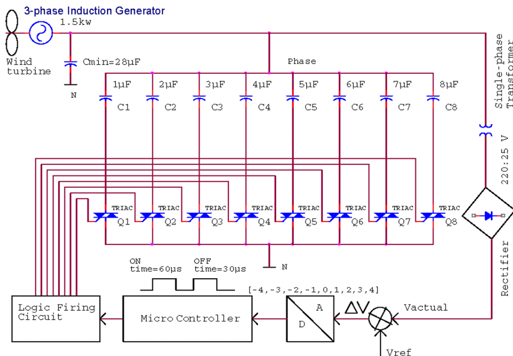
Рисунок 3.6 – Дискретное регулирование емкостей возбуждения АГ
