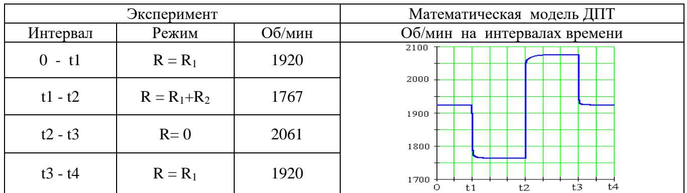
Рисунок 4.6 – Изменение числа оборотов ДПТ при разных величинах сопротивлений в цепи якоря
