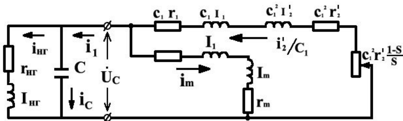
Рисунок 2.2 – Схема замещения АГ с линейной L_m
