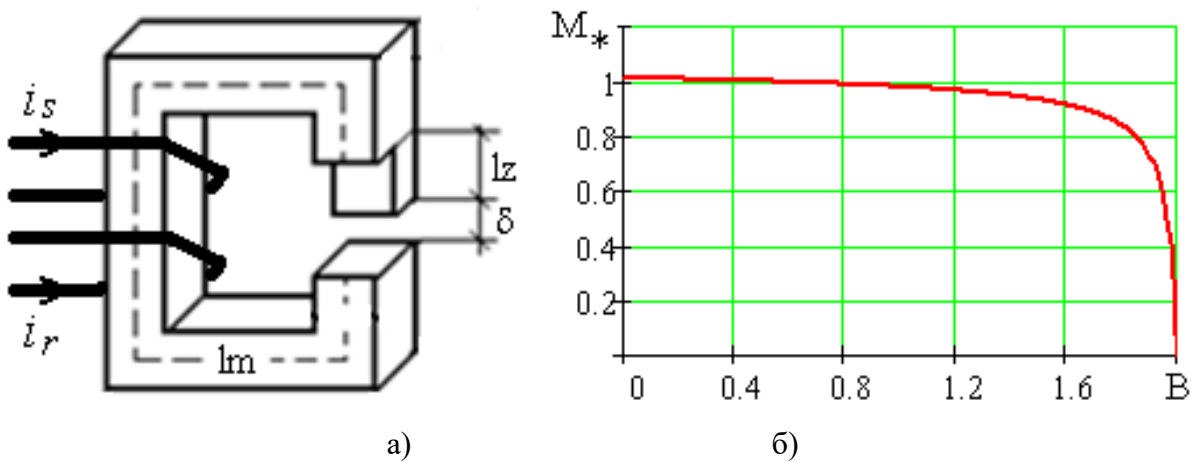
Рисунок 2.9 – Упрощенная модель неоднородного магнитопровода с зазором (а) и расчетная зависимость изменения взаимоиנדукции между обмотками
