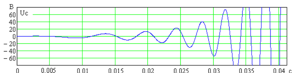
Рисунок 2.7 – Процесс нарастания частоты и амплитуды напряжения на емкости АГ при самовозбуждении
