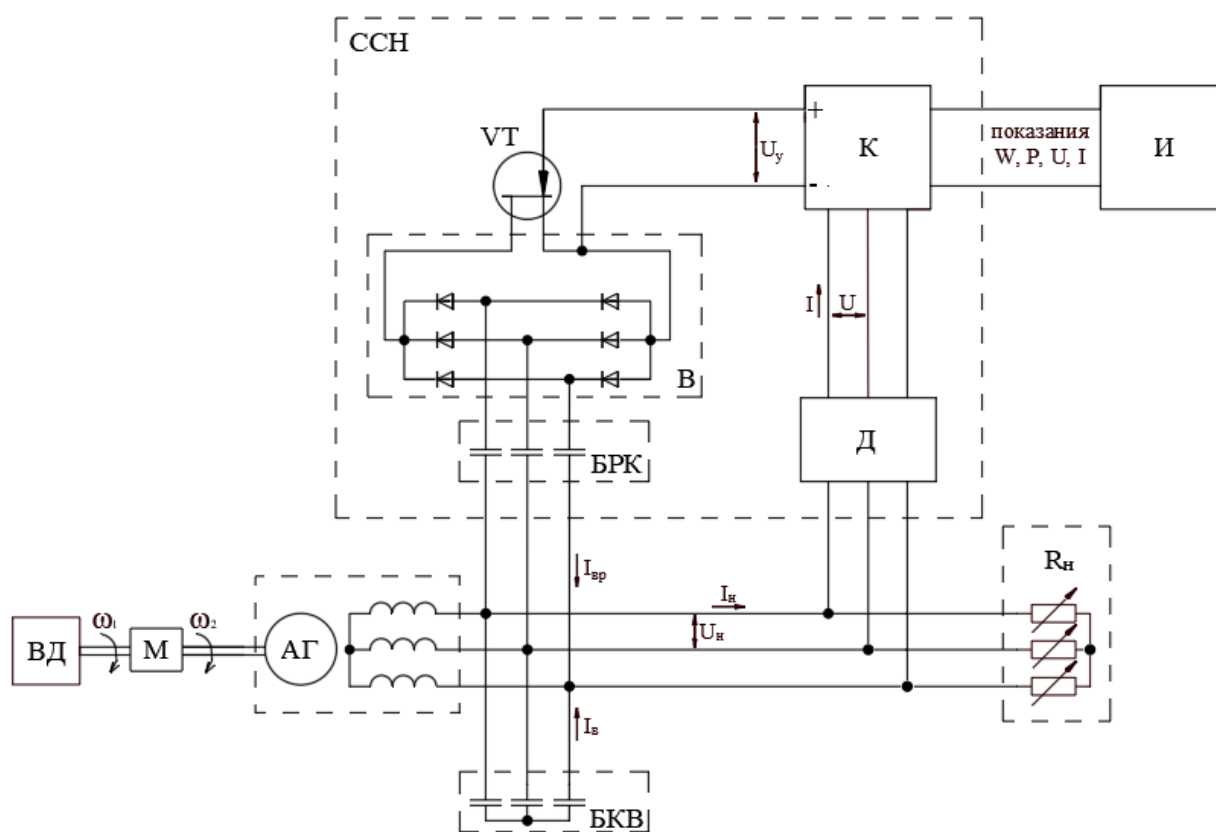
Рисунок 3.15 – Функциональная схема устройства стабилизации напряжения ветроэнергетической установки
