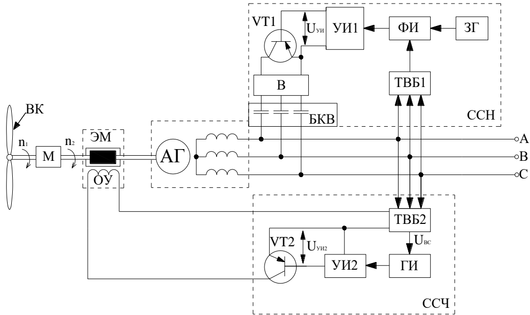
Рисунок 1.17 – Устройство стабилизации напряжения и частоты ветроэнергетической установки
