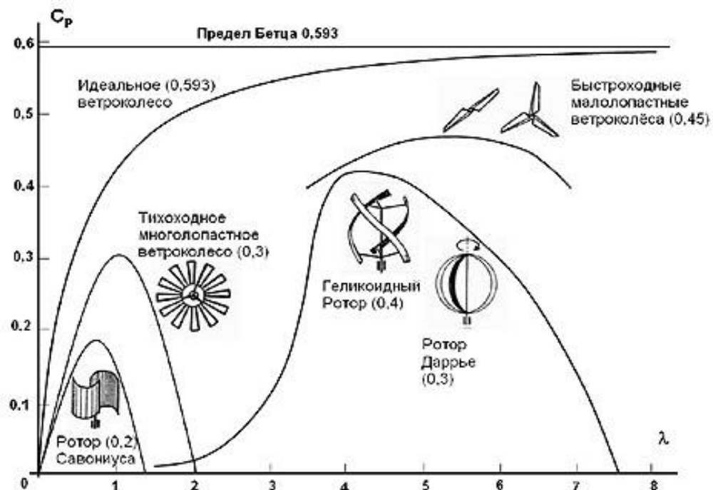
Рисунок 1.9 – Зависимости коэффициента использования энергии ветрового потока от быстроходности различных ветродвигателей (аэродинамические характеристики ветродвигателей)
