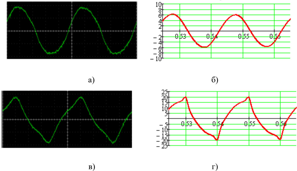
Рисунок 4.2 – Ток фазы АД при подаче напряжения 220 В (а – опыт, б – расчет) и при подаче напряжения 380 В (в – опыт, г – расчет)
