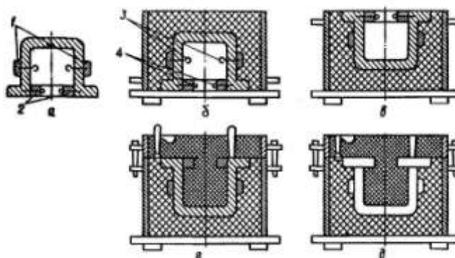
Рисунок 1 – Формовка по модели с отъемными частями.
