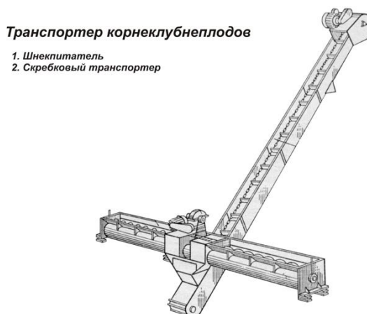
Рисунок 1 – Транспортер корнеклубнеплодов
