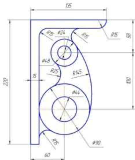
Рисунок 1 Вариант 1 Кронштейн
