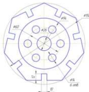
Рисунок 4 Вариант 4 Пластина
