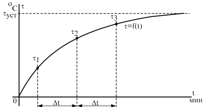
Рисунок 12.4. Кривую нагрева электродвигателя
