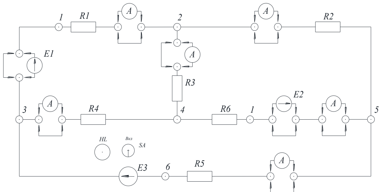
Рисунок 2.2 –Исследуемая схема
