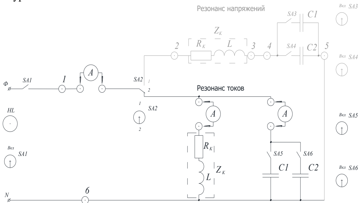
Рисунок 4.2 – Исследуемая схема
