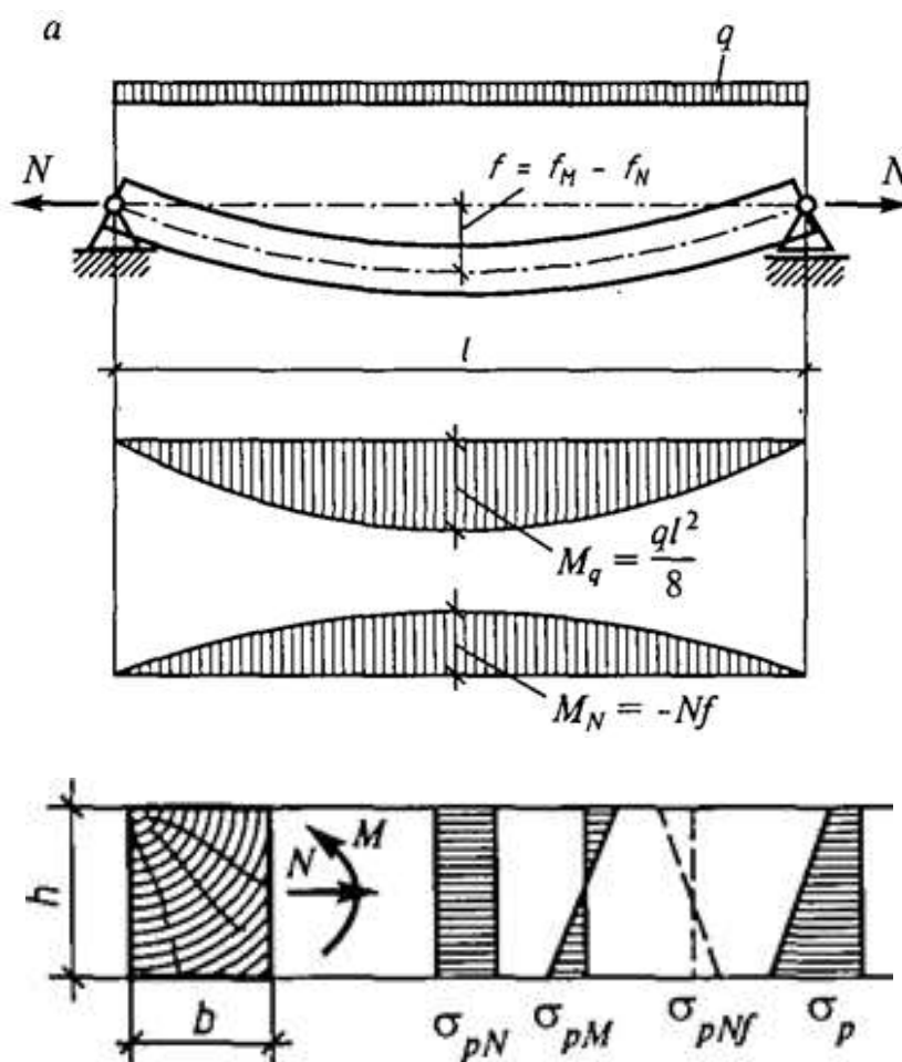
Рисунок 2.6 – Растянуто-изгибаемый элемент:
