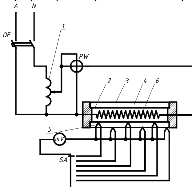
Рисунок 2 – Установка для определения коэффициента теплопроводности 6 ПОРЯДОК ПРОВЕДЕНИЯ ЭКСПЕРИМЕНТА
