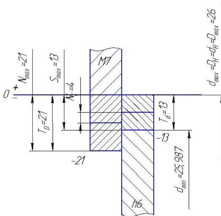
Рисунок 1– Схемы полей допусков посадки \frac{M7}{h6} Ø26
