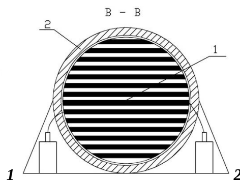
Рисунок 1. – озонатор с предварительной подготовкой воздуха (разрез вид сбоку);
