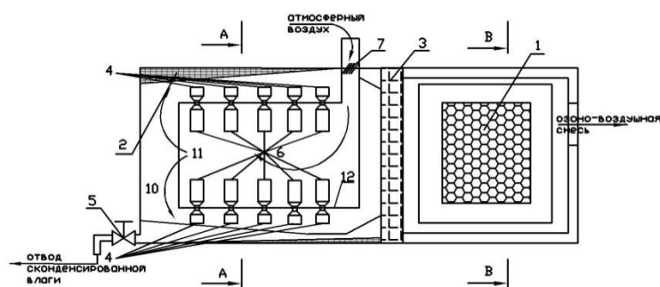
Рисунок 1. – озонатор с предварительной подготовкой воздуха (разрез вид сбоку);
