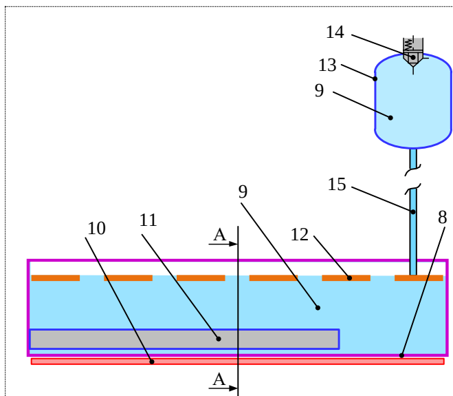
Рисунок 3 – Устройство поилки для пчел: вид с боку
