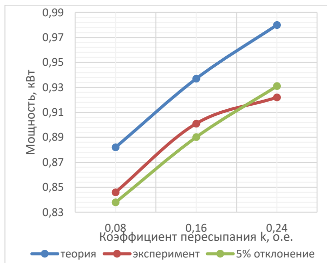
Рисунок 13 – график сходимости теоретических и экспериментальных результатов
