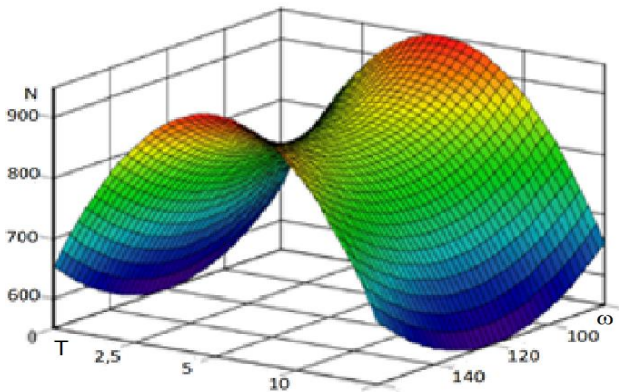
Рисунок 10 - Поверхность зависимости однородности от количества отверстий в мешалке и времени смешивания и его двумерное сечение
