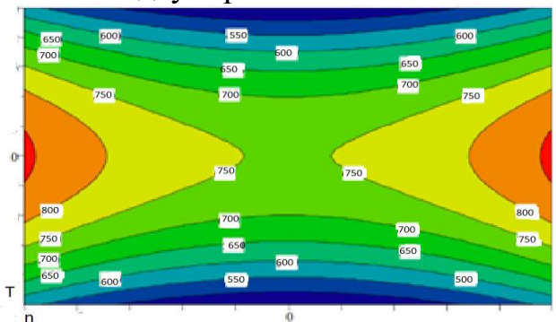
Рисунок 11 - Поверхность зависимости производительности от частоты вращения и времени смешивания и его двумерное сечение
