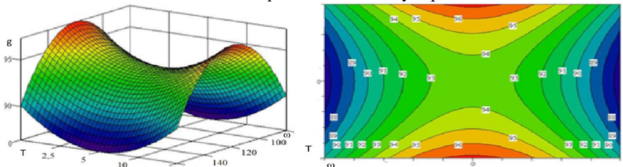
Рисунок 7- Поверхность зависимости однородности от количества отверстий в мешалке и времени смешивания и его двумерное сечение
