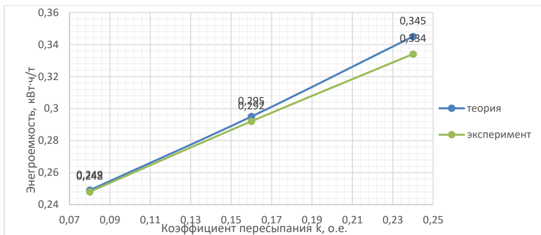
Рисунок 14 – График зависимости энергоёмкости процесса смешивания от коэффициента пересыпания k
