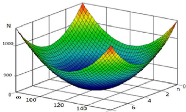
Рисунок 9 - Поверхность зависимости однородности от количества отверстий в мешалке и частоты её вращения и его двумерное сечение
