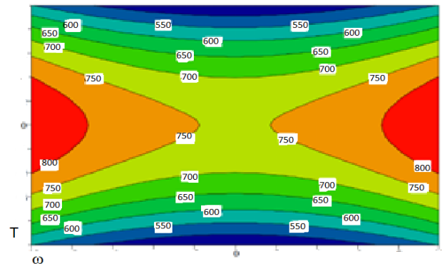
Рисунок 10 - Поверхность зависимости однородности от количества отверстий в мешалке и времени смешивания и его двумерное сечение
