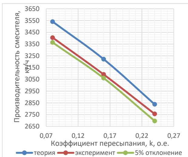
Рисунок 12 – график сходимости теоретических и экспериментальных результатов
