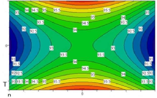
Рисунок 8 - Поверхность зависимости производительности от частоты вращения и времени смешивания и его двумерное сечение
