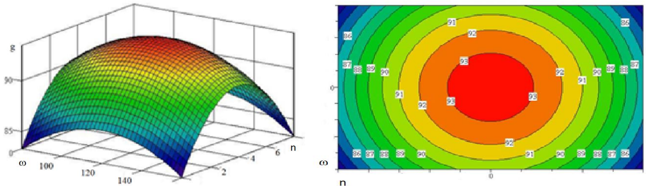
Рисунок 6 - Поверхность зависимости однородности от количества отверстий в мешалке и частоты её вращения и его двумерное сечение
