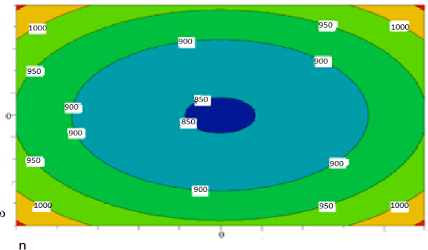
Рисунок 9 - Поверхность зависимости однородности от количества отверстий в мешалке и частоты её вращения и его двумерное сечение
