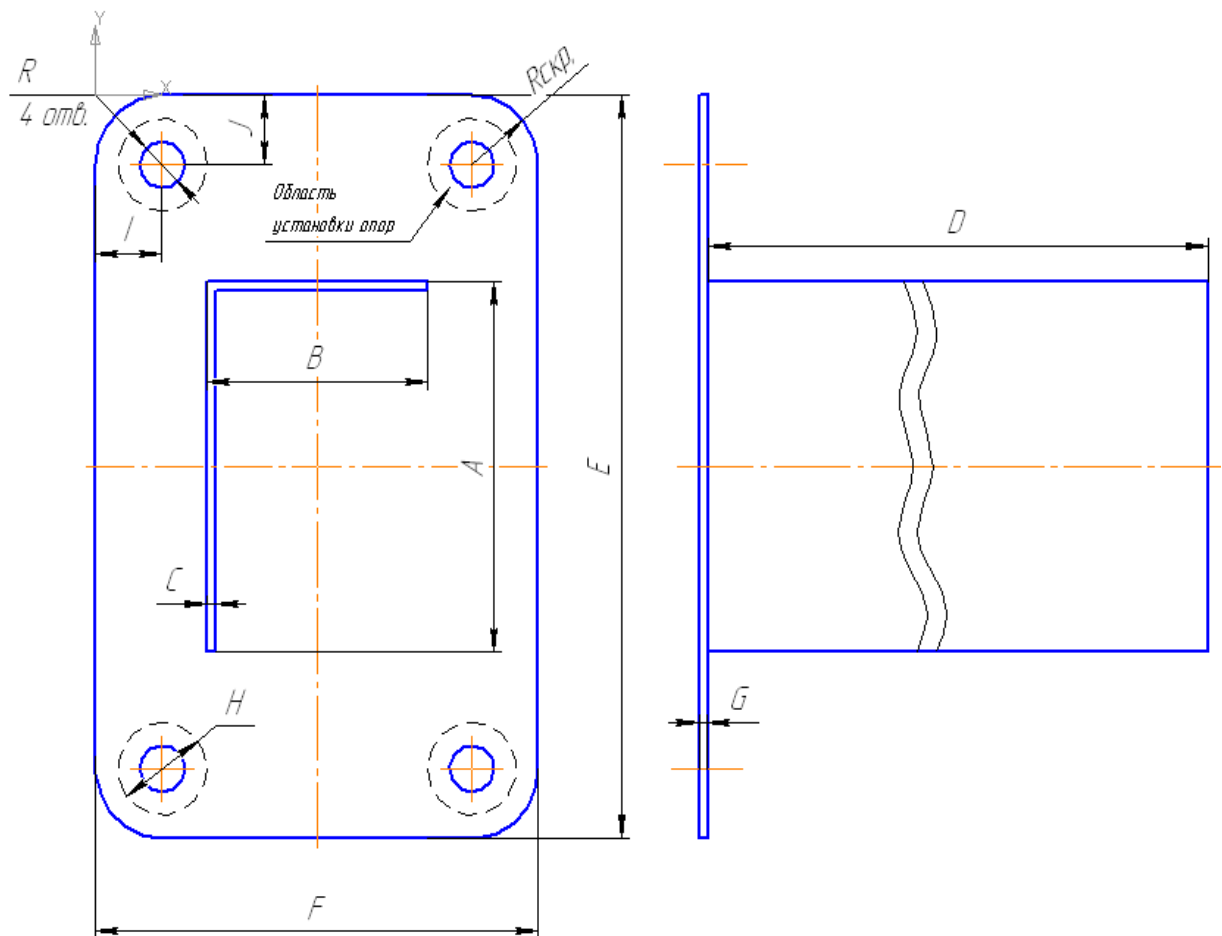
Рисунок 2 Чертёж кронштейна для самостоятельного выполнения расчёта.
