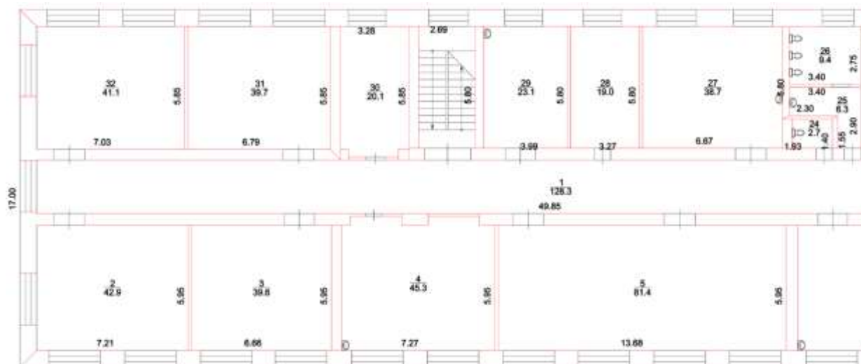
План помещения №5.
