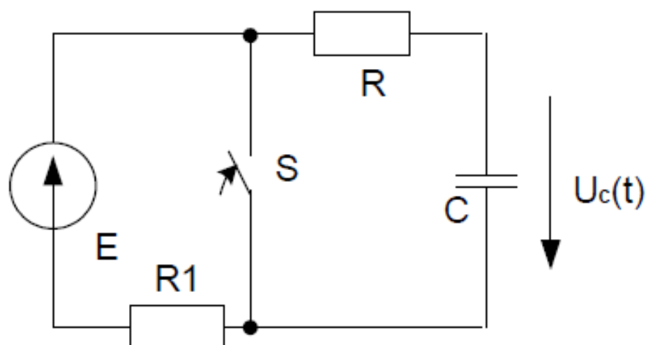
Рисунок 3 – Принципиальная схема
