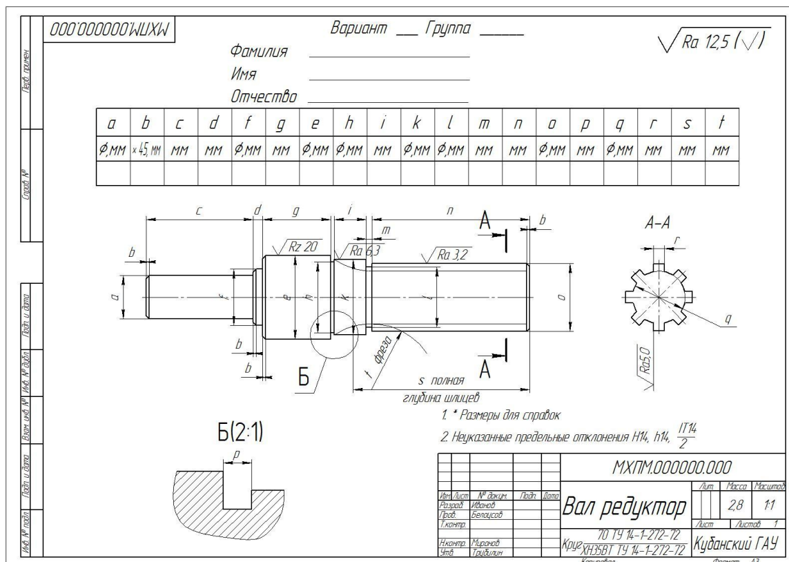
Рисунок 5 – типовой чертеж детали «ВАЛ РЕДУКТОР»
