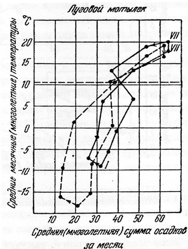
Рисунок 7 – Климодиаграммы оптимума для лугового мотылька в Европейской части России (сплошная линия) и в Сибири (прерывистая линия) (по Бей-Биенко, 2008)
