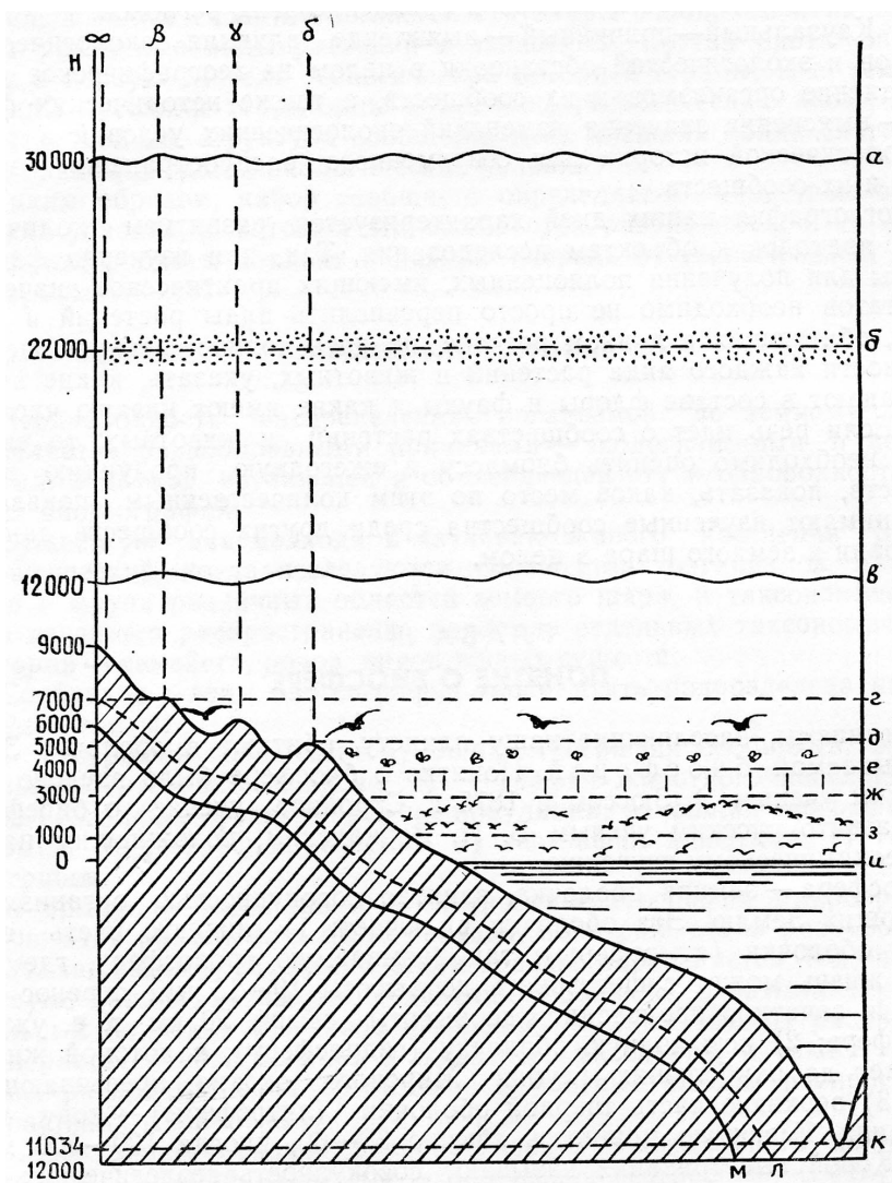
Рисунок 1 – Пределы биосферы (по Воронову, 1987):
