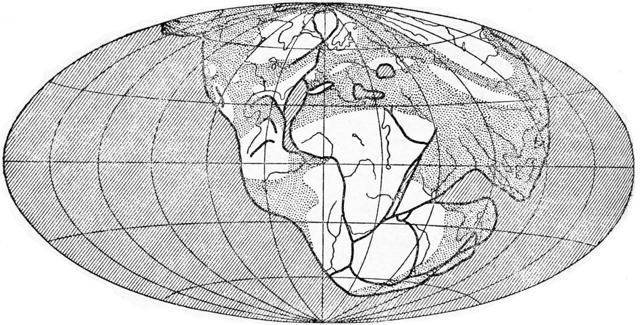
Рисунок 13 – Структура земной коры в каменноугольный период (по Пузанову, 1938)
