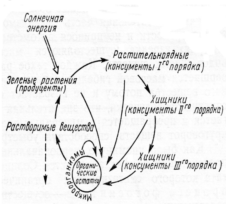
Рисунок 2 – Круговорот вещества в биосфере (по Воронову, 1987):
