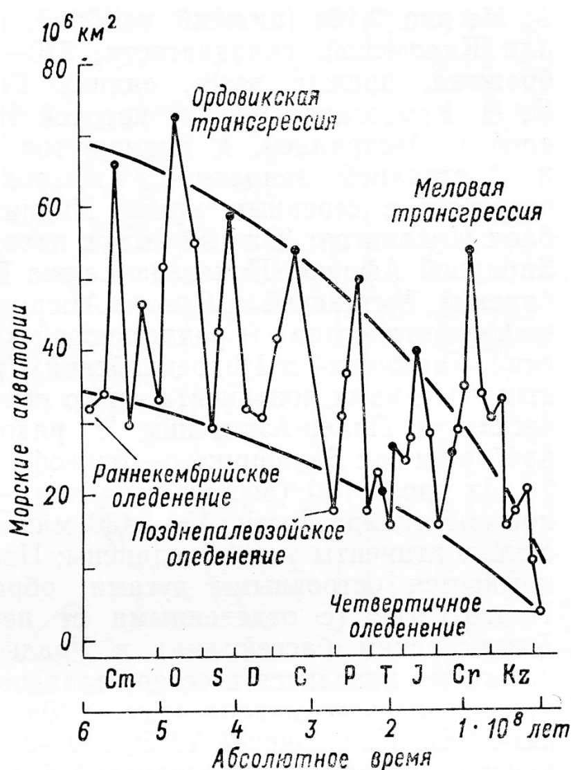
Рисунок 11 – Изменения суммарной площади покрытых морями территорий современных континентов (по Монину, Шишкову, 1979)
