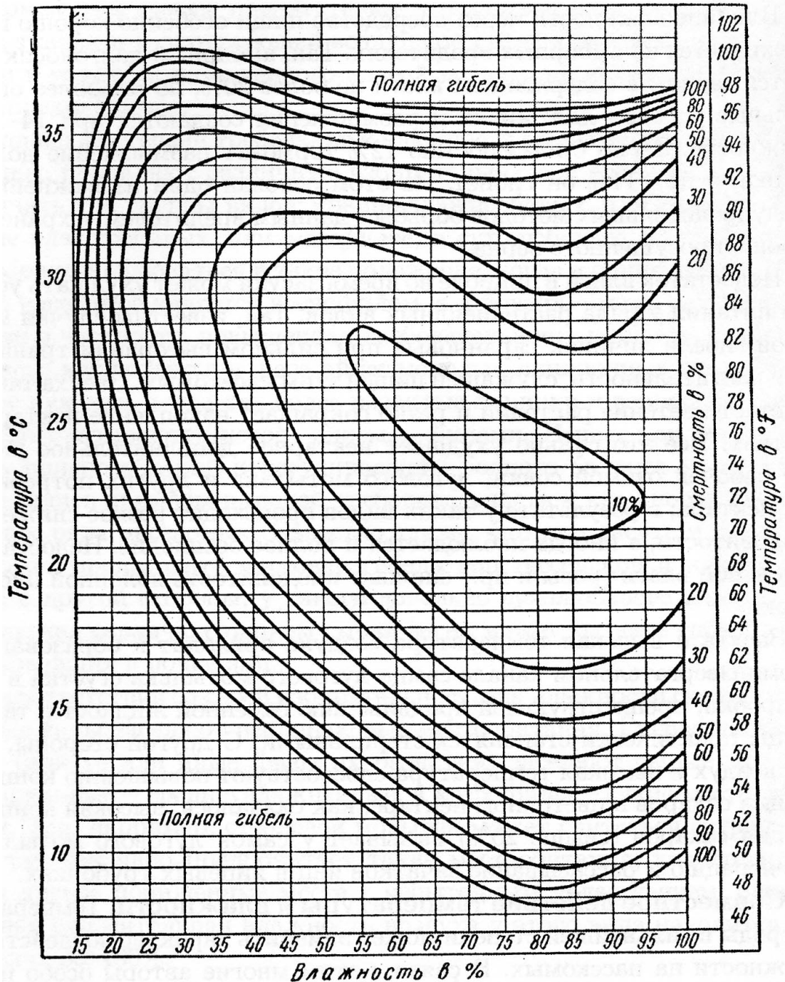
Рисунок 6 – Гигротермограмма развития куколки яблонной плодовой жоржки (по Бей-Биенко, 2008):
