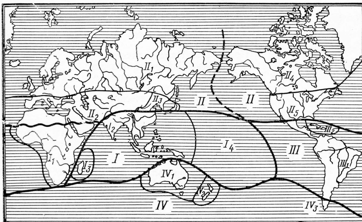
Рисунок 16 – Фаунистические области суши (по Лопатину, 1989):
