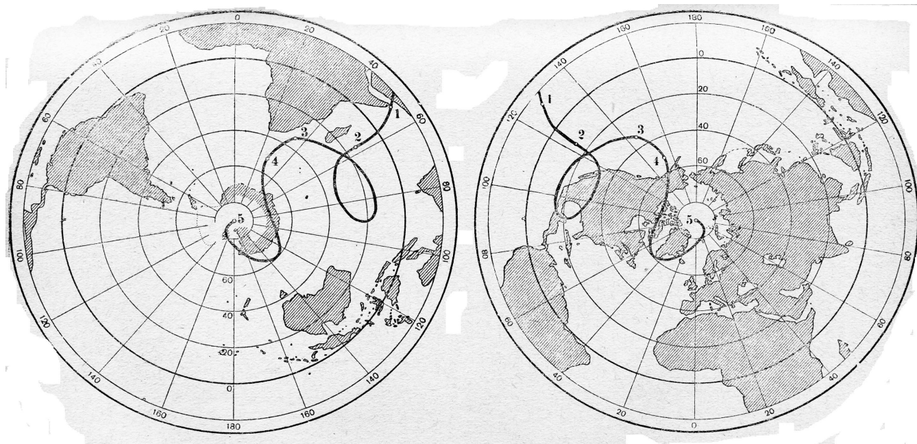
Рисунок 15 – Пути северного и южного полюсов в течение геологического времени (по Пузанову, 1938):
