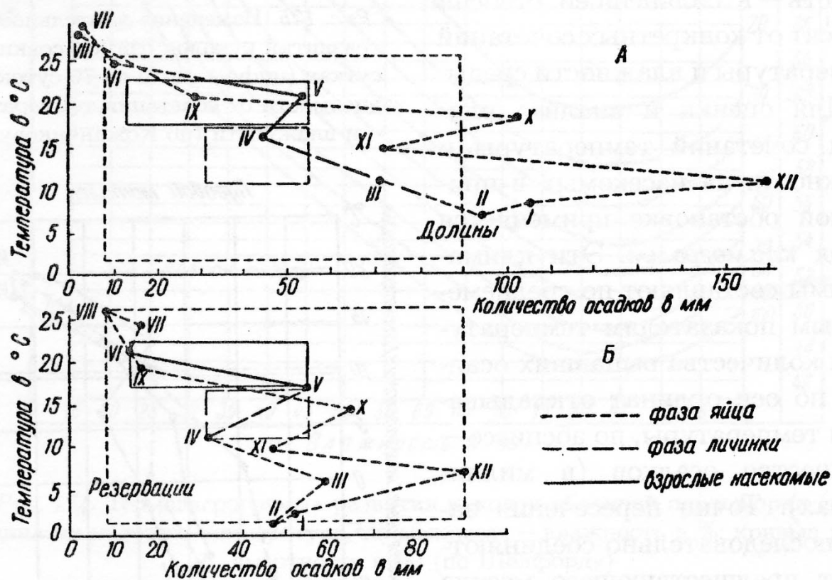
Рисунок 8 – Биоклимодиграма Уварова для мароккской саранчи (по Бей-Биенко, 2008):
