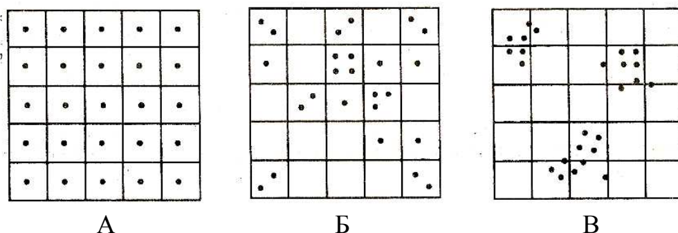
Рисунок 4 – Типы пространственного распределения особей в популяциях (по Шилову, 1997):
