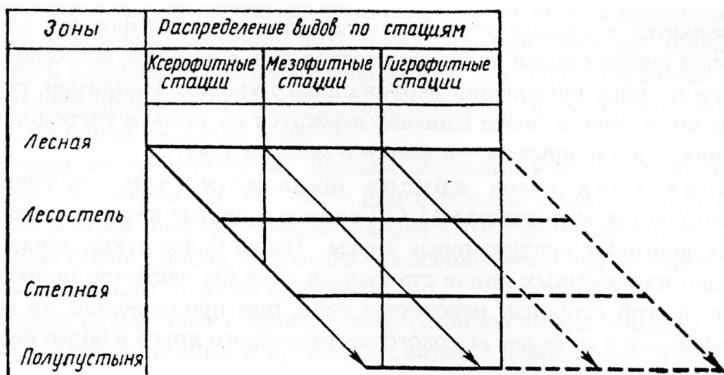
Рисунок 10 – Диаграмма зональной смены станций (по Бей-Биенко, 2008)
