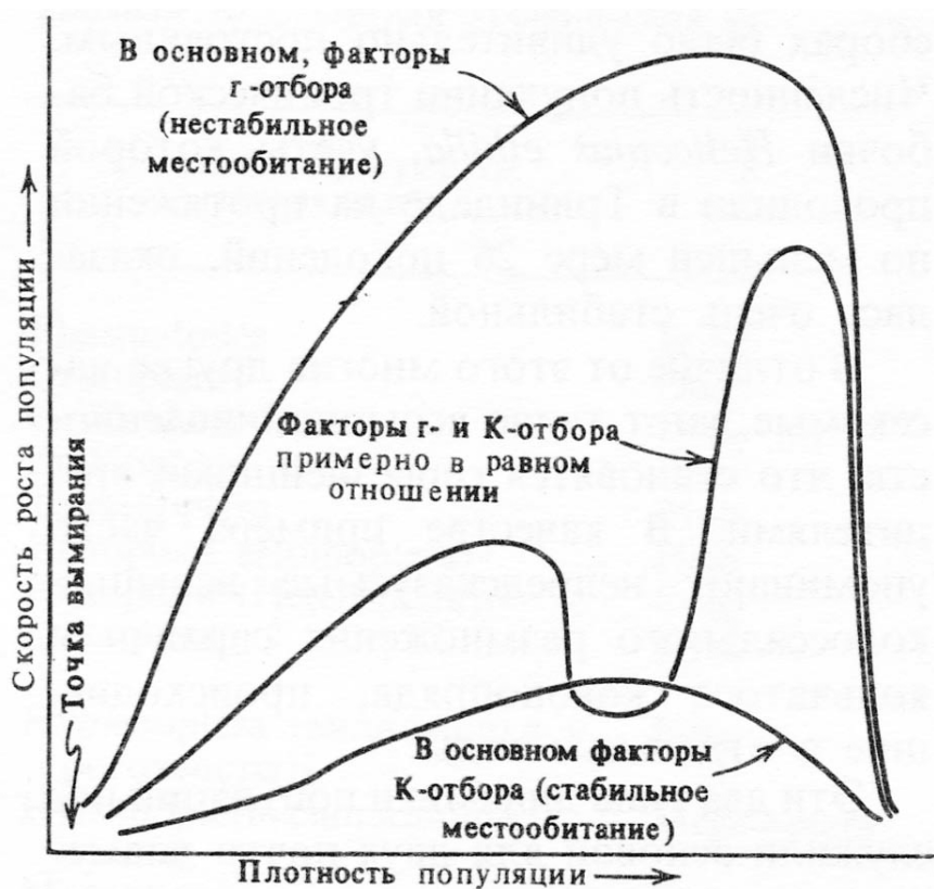
Рисунок 3 – Модели трех различных типов роста численности и плотности популяций (по Г. Росс, Ч. Росс, Д. Росс, 1985):
