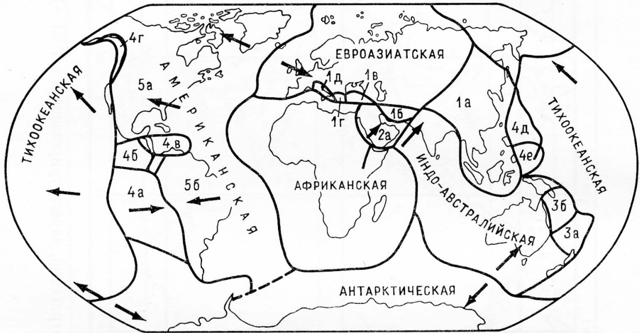
Рисунок 12 – Литосферные плиты (по Мониному, Шишкову, 1979):
