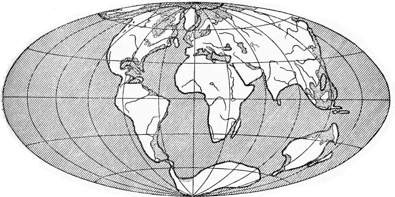
Рисунок 14 – Структура земной коры в четвертичный период (по Пузанову, 1938)
