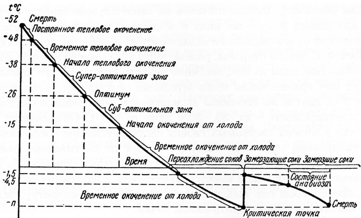
Рисунок 5 – Кривая Бахметьева, характеризующая изменение состояния насекомого под воздействием температуры среды (по Бей-Биенко, 2008)
