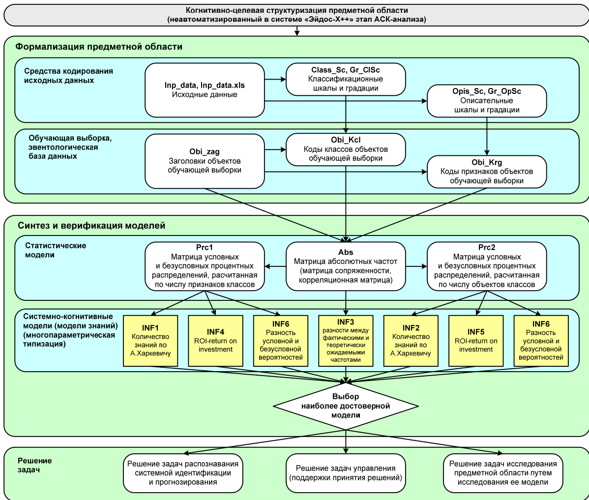
Рисунок 1. Этапы АСК-анализа
