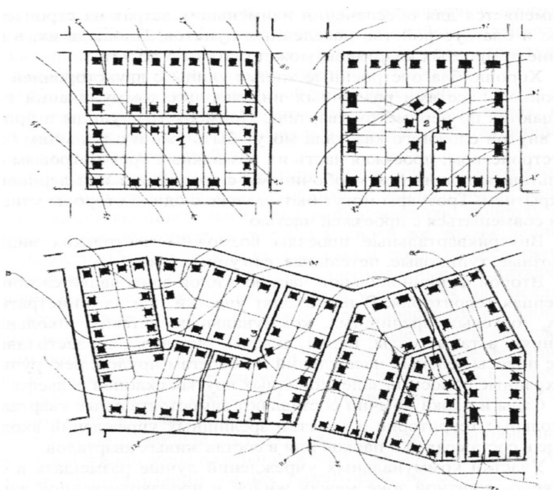
Рисунок 13 – Сложные кварталы участковой застройки: 1 – со сквозным проездом; 2 – с тупиковым проездом; 3 – с петельным проездом; 4 – с фигурным проездом
