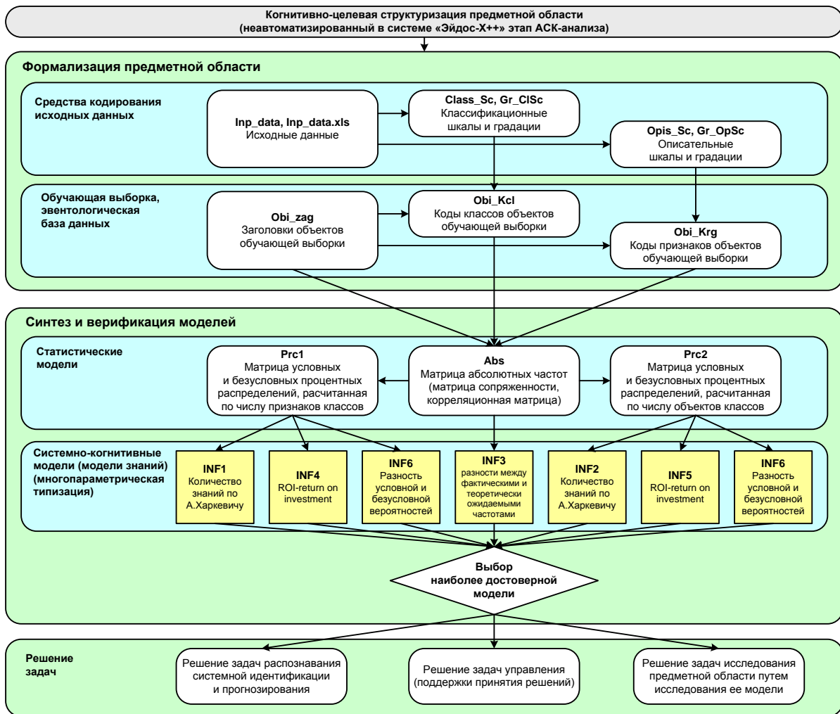
Рисунок 1. Этапы АСК-анализа
