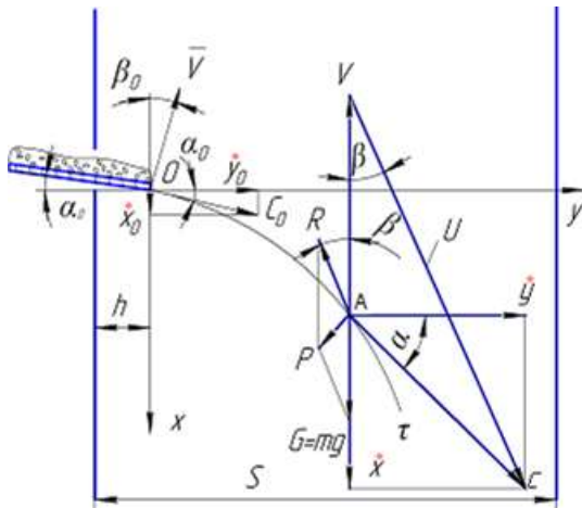
Рисунок 2 – Схема скоростей перемещения и сил, действующих на j -тый компонент семян крупноплодного подсолнечника в воздушном потоке вертикального канала
