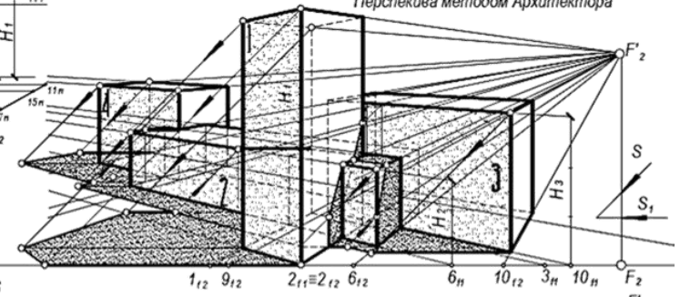
ОБРАЗЕЦ выполнения эюра "Перспектива методом Архитектора"
