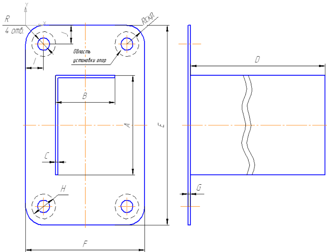
Рисунок 2 Чертеж кронштейна для самостоятельного выполнения расчёта.
