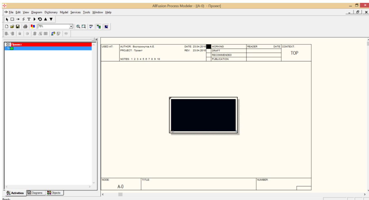
Рисунок 4 – Интерфейс приложения
